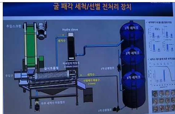
<수산부산물 전처리시설 예시>
